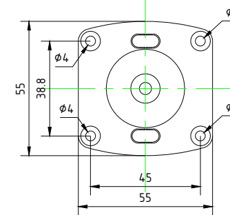
ВИД СПЕРЕДИ / FRONT VIEW
