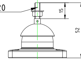
ВИД СПЕРЕДИ / FRONT VIEW
